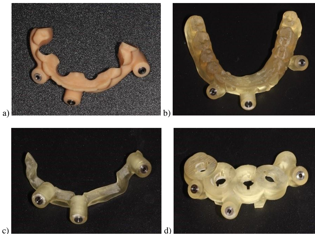
Рис. 11. Напечатанные позиционер (a) и шаблоны: позиционирующий (b), костный (c), навигационный (d)
